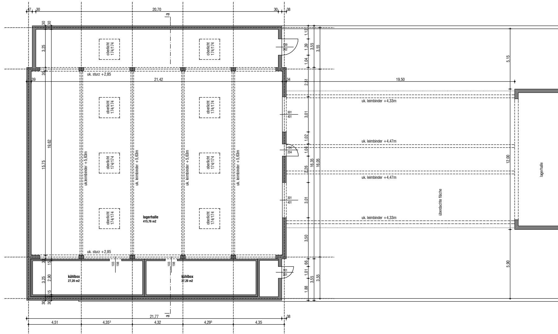
lageplan m 1/200
