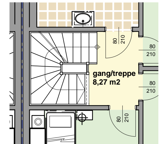
TREPPE bei Ausführung STUDIO
